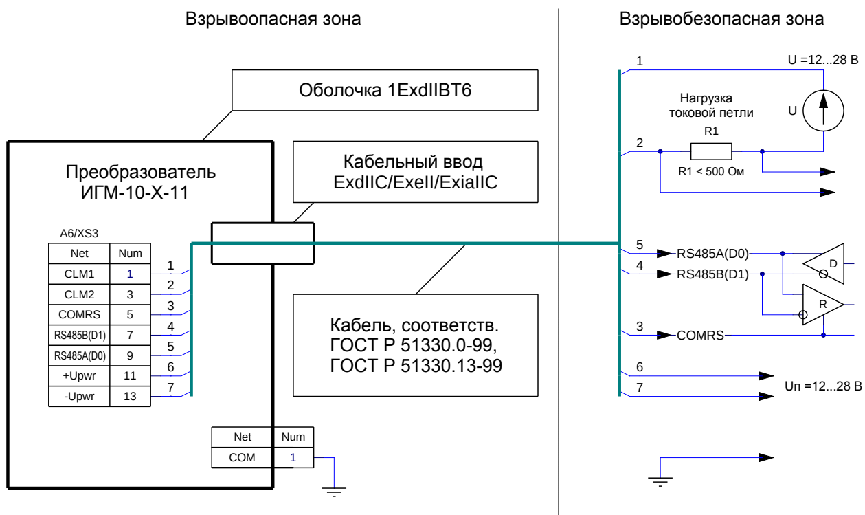
Рисунок Б.3 – Схема подключения преобразователя ИГМ-10-Х-11 (с кабельным вводом)
