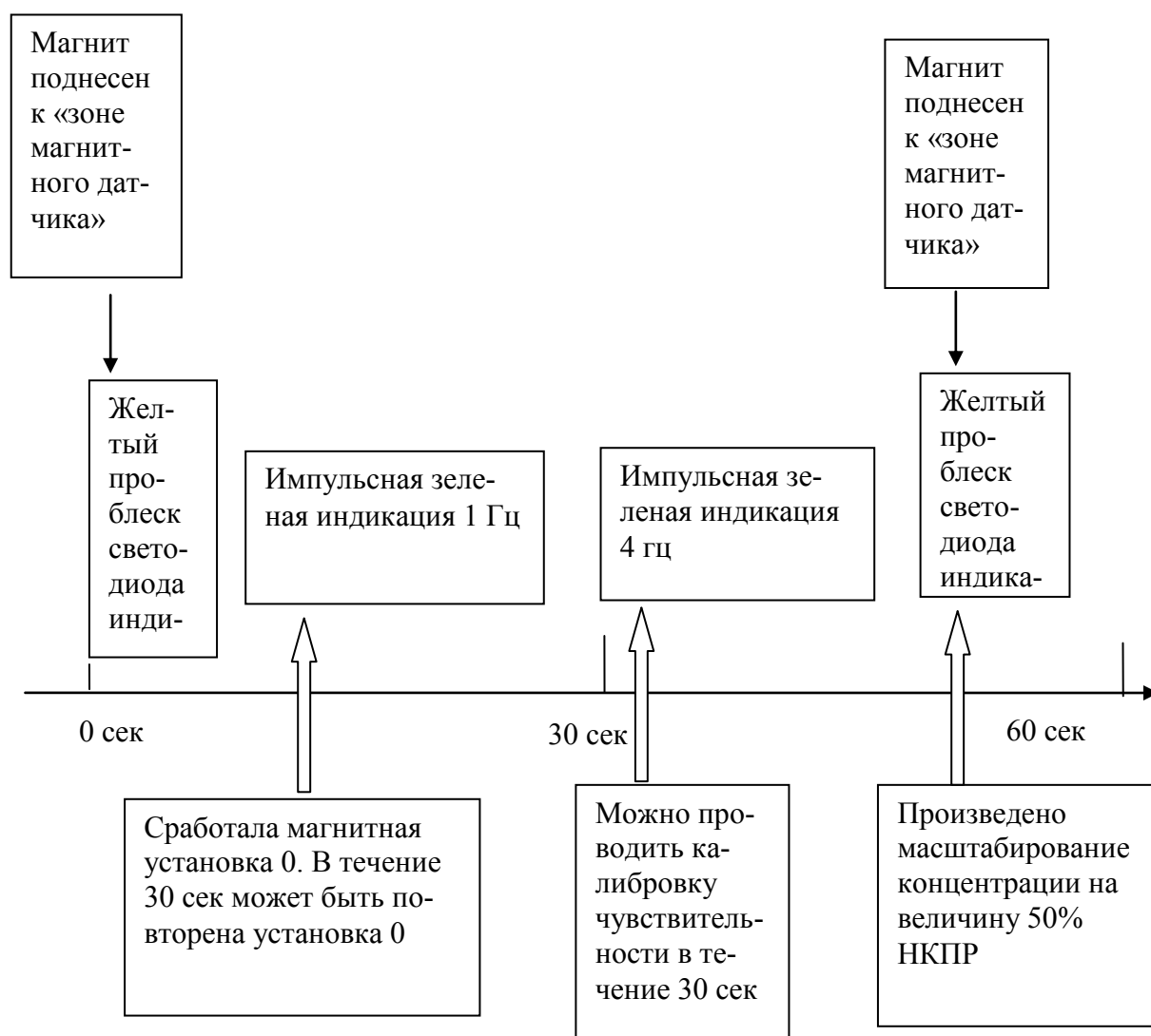
Рис. 3.1. Диаграмма калибровки
