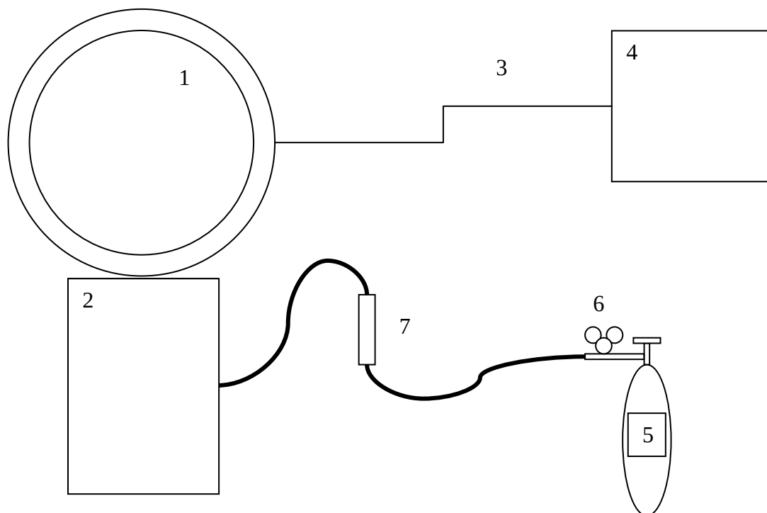
Рисунок 3.2 –схема калибровки.
